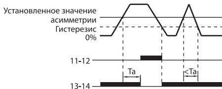
Рисунок 7. Схема работы реле PH 12 при асимметрии фаз
