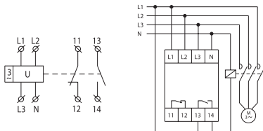
Рисунок 3. Схема подключения реле PH 12 к электрической сети
