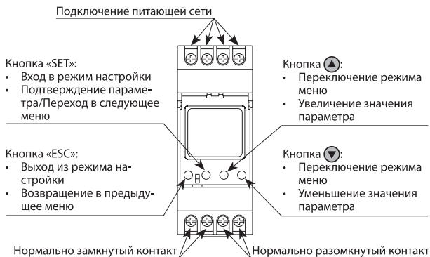
Рисунок 4. Внешний вид управляющих элементов реле RH 12
