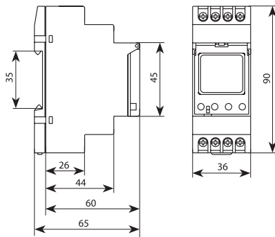
Рисунок 2. Габаритные и установочные размеры реле напряжения серии PH 12, мм
