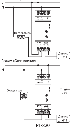
Рисунок 2. Схемы подключения реле
