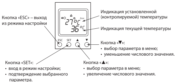
Рисунок 6. Показания дисплея реле PT-820M
